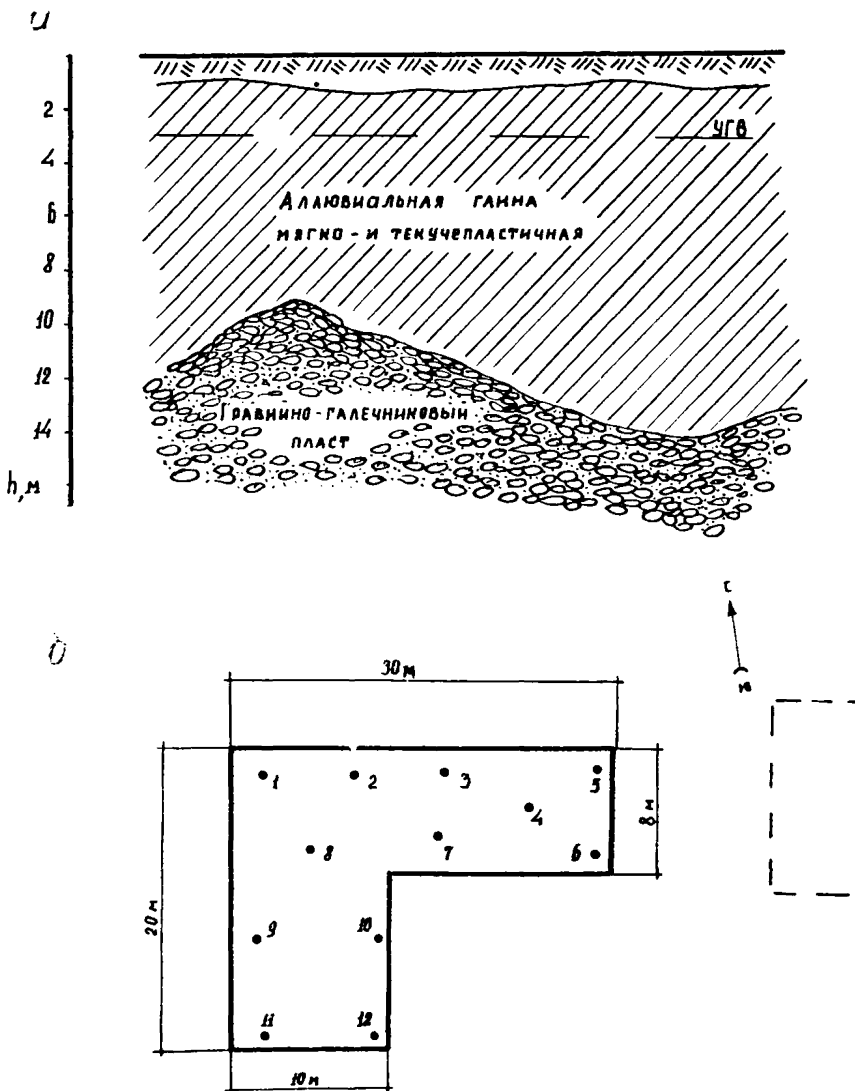
Рис.2. Исходные данные к примеру 2: а-литологический разрез площадки; б-расположение точек зондирования.
