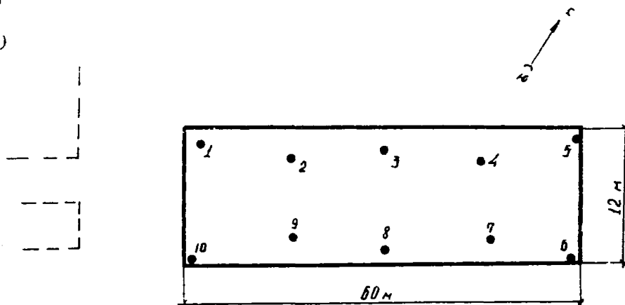
Рис. I. Исходные данные к примеру I: а-литологический разрез площади; б-расположение точек зондирования
