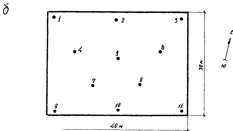
Рис.3. Исходные данные к примеру 3 приложения I и к приложению 2 : а-литологический разрез площадки; б-расположение точек зондирования
