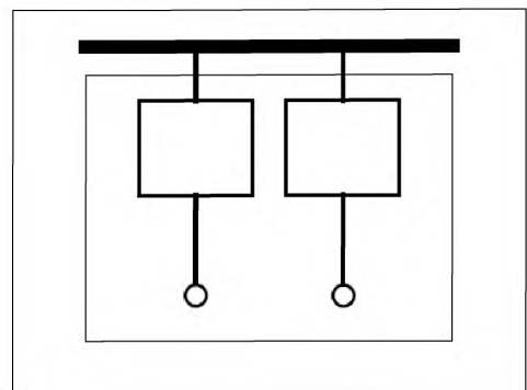
Вид внутреннего разделения 2б: выводы отделены от сборных шин
