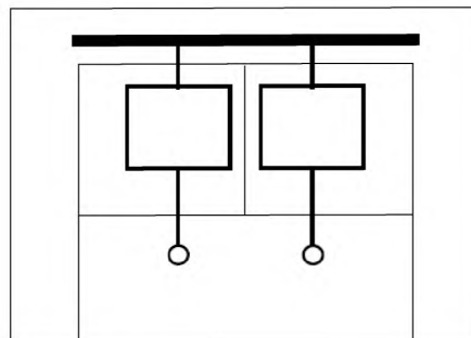
Вид внутреннего разделения 3b: выводы и внешние проводники отделены от сборных шин
