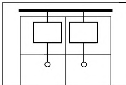
Вид внутреннего разделения 4b: выводы и соединенный с ними функциональный блок находятся в разных отсеках
