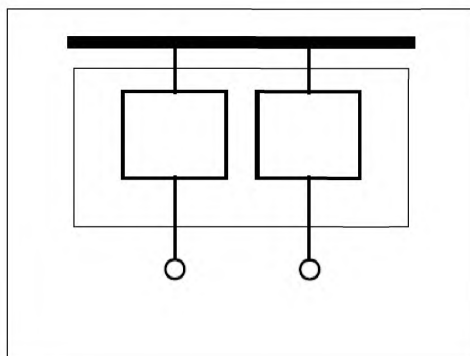
Вид внутреннего разделения 2а: выводы не отделены от сборных шин
