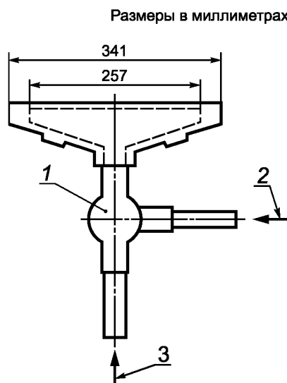
Рисунок 5а — Одиночная горелка, используемая при стандартной лестнице
