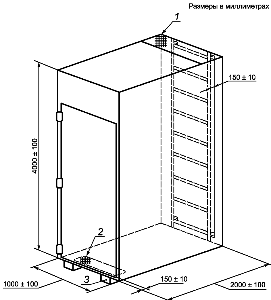
Рисунок 1а — Испытательная камера
