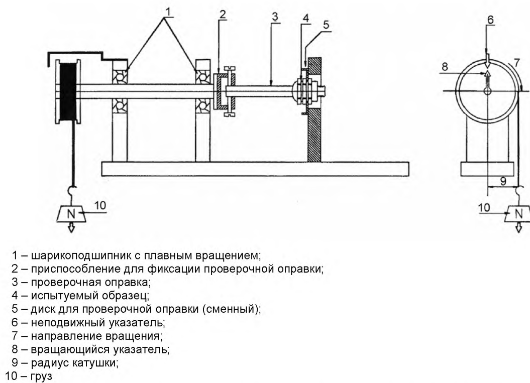
Рисунок 9 – Типичное устройство для испытания стойкости к растяжению скручиванием
