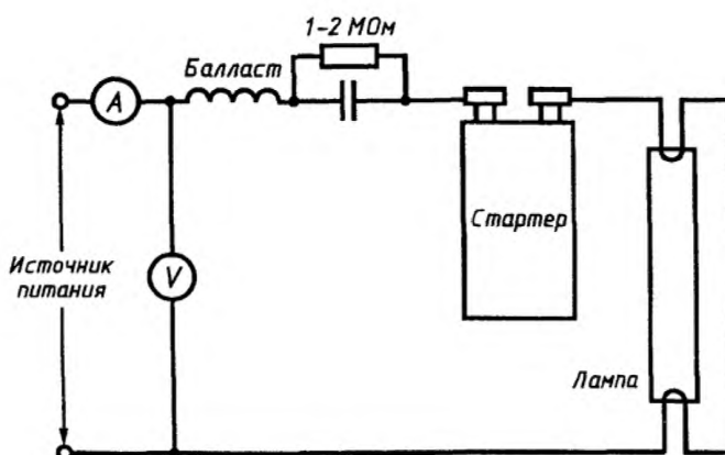
Рисунок 7 – Схема испытания стартеров на зажигание
