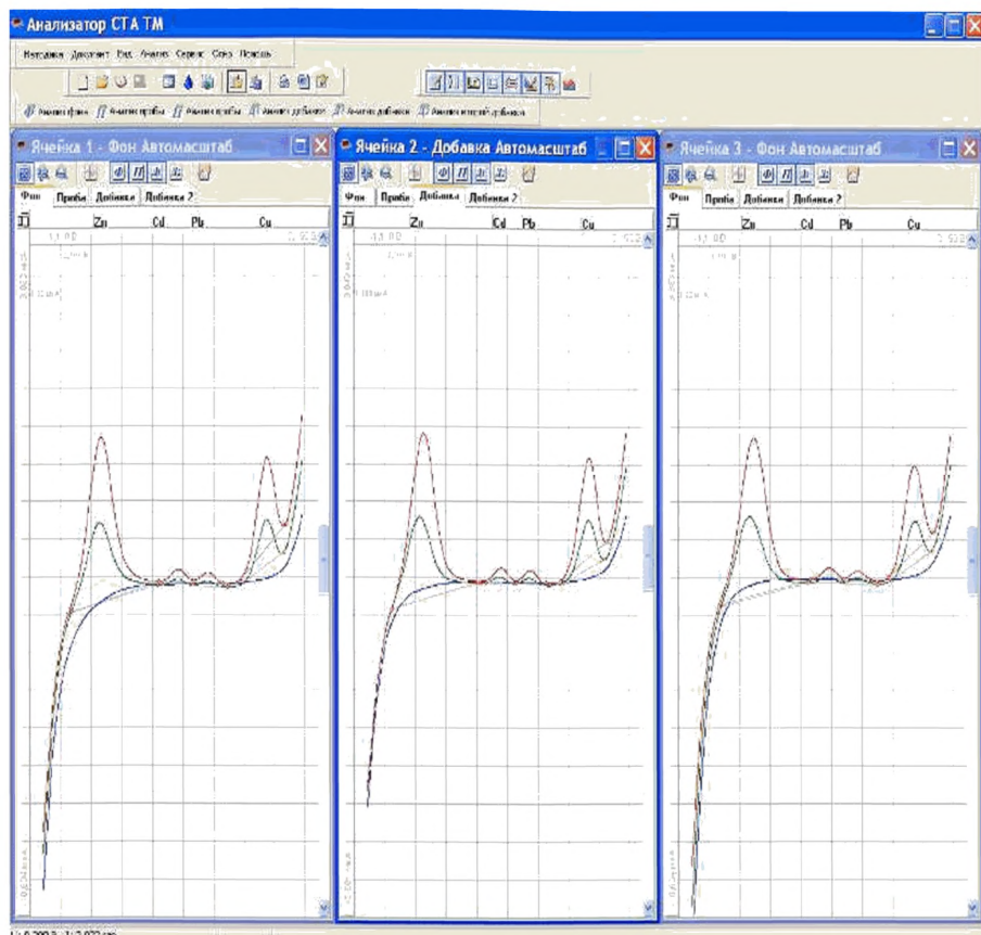
Рисунок 4. Вольтамперограммы цинка, кадмия, свинца и меди (одновременное определение) в растворе фоновое электролита, пробы и пробы с добавками АС элементов
