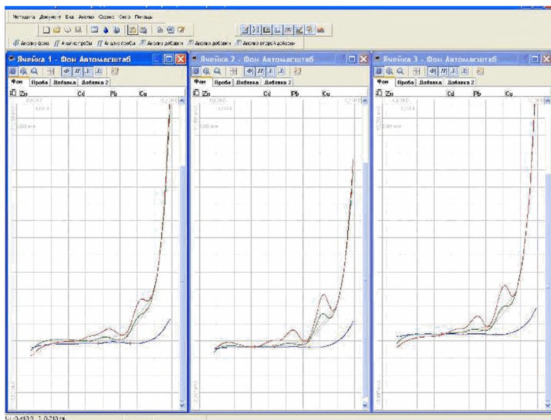
Рисунок5. Вольтамперограммы кадмия, свинца и меди (с отсечением цинка) в растворе фоновго электролита, пробы и пробы с добавками АС элементов
