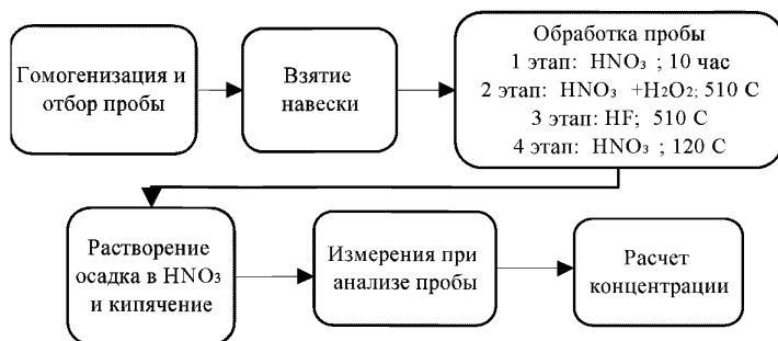
Рисунок 1. Основные этапы анализа проб угля на содержание серебра
