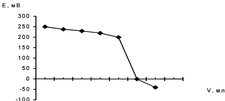
Рисунок 2. Вид кривой потенциометрического титрования \text{Ag}^+ раствором \text{KJ}
