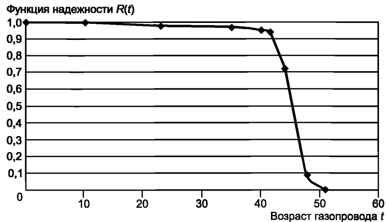
Рисунок Б.1 — График эмпирической функции надежности R(t)
