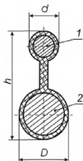
1 – трос; 2 – сердечник кабеля; d – диаметр изолированного троса; D – диаметр кабеля; h – высота кабеля
