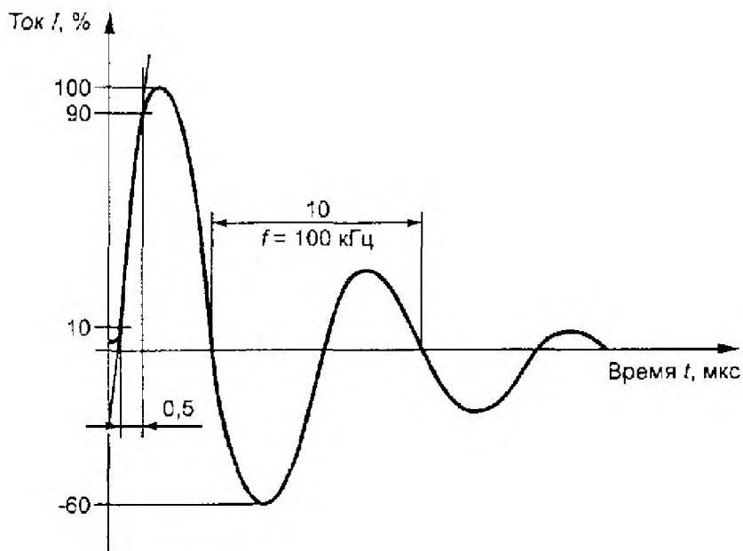
Рисунок В.4 — Волна тока 0,5 мкс/100 кГц
