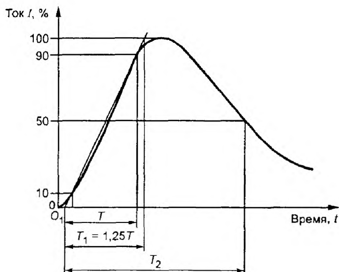
Рисунок В.6 — Волна импульсного тока 8/20 мкс
