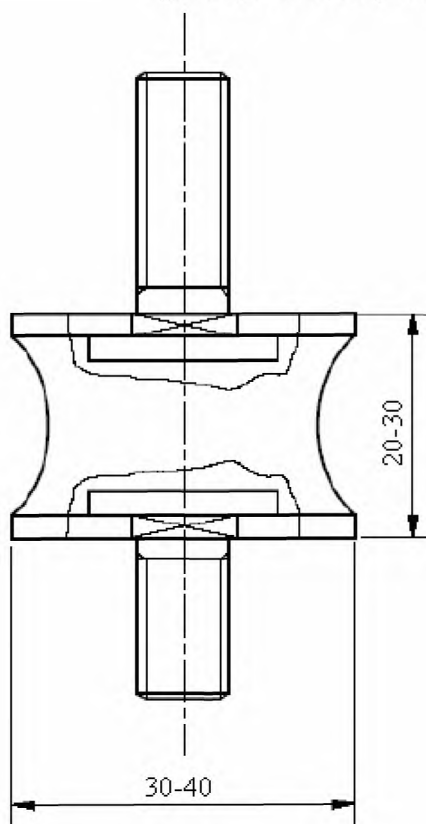
Рисунок 4 – Типовая резиновая втулка для крепления испытательной лестницы
