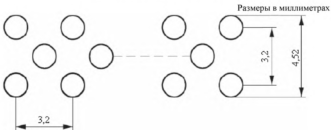
Рисунок 5 – Поверхность горелки
