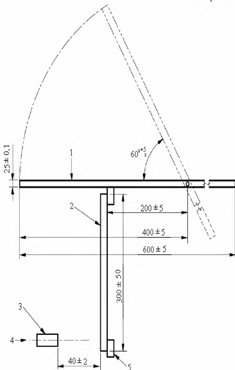
1 - ударное устройство; 2 - панель; 3 - газовая горелка; 4 - центральная линия передней поверхности горелки; 5 - опорная рамная конструкция. Рисунок 3 – Оборудование для испытания (вид сбоку)
