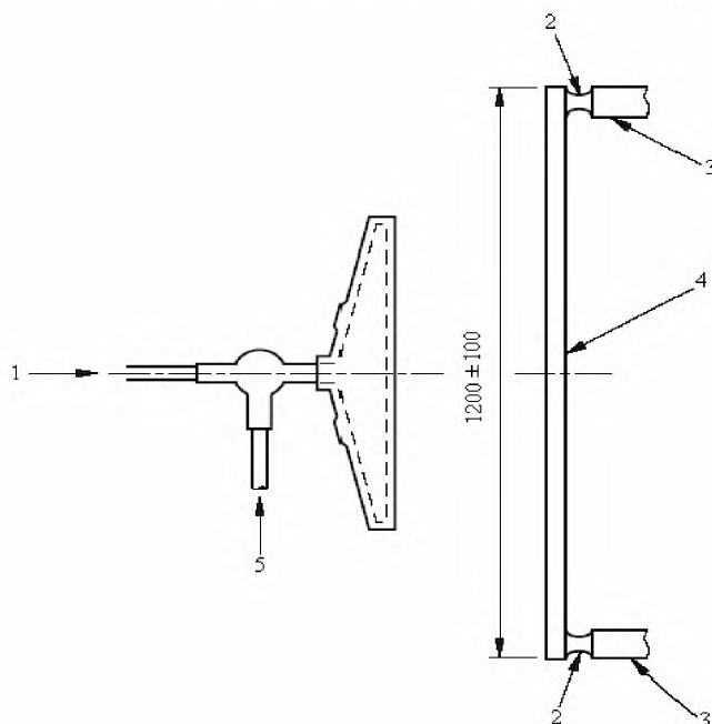
Рисунок 2 – Рекомендуемый метод установки металлического корпуса к испытательной лестнице
