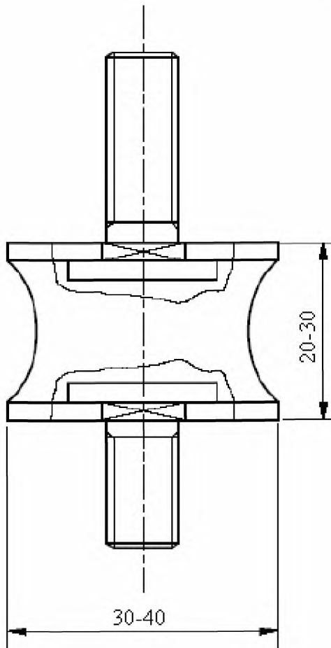
Рисунок 5 – Типовая резиновая втулка для поддержки испытательной лестницы
