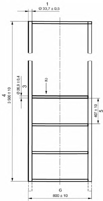
Рисунок 4б – Широкая лестница
