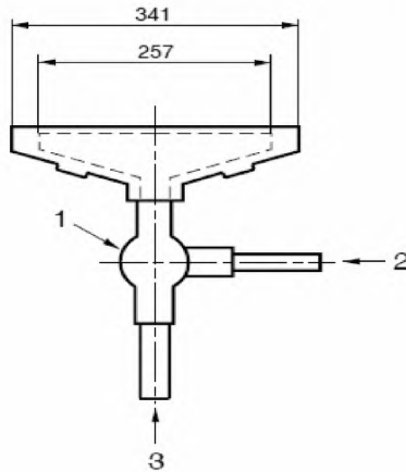
Рисунок 5а – Одиночная горелка, используемая при стандартной лестнице
