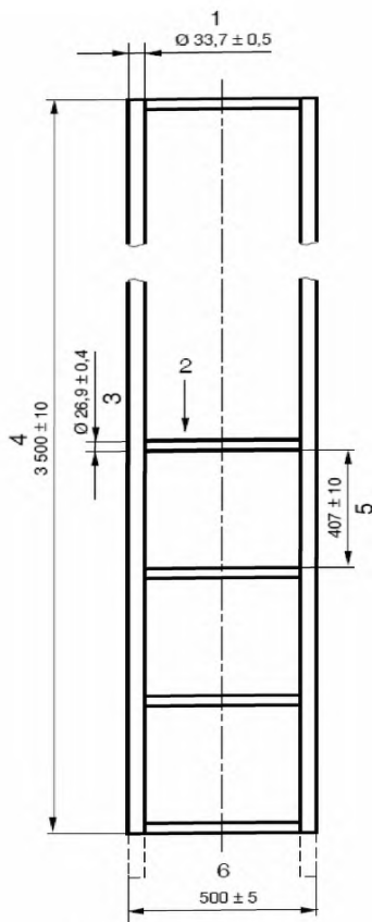
Рисунок 4а – Стандартная лестница
