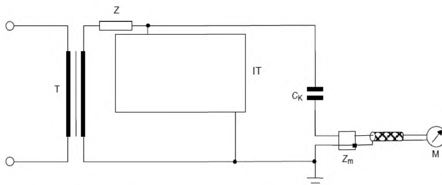
Рисунок 6 — Альтернативная схема измерения частичных разрядов
