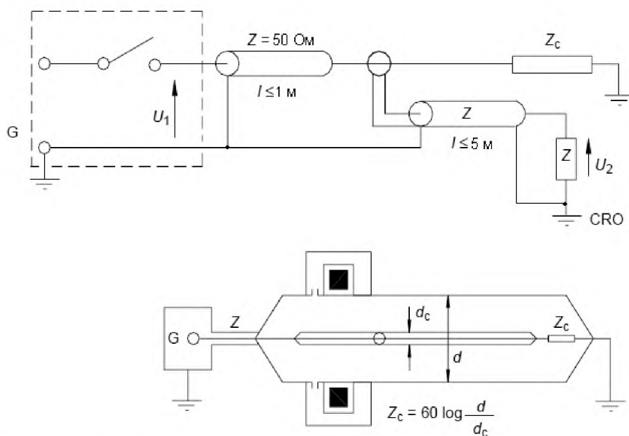
Рисунок 9 — Измерение передаваемых перенапряжений. Общая структурная схема
