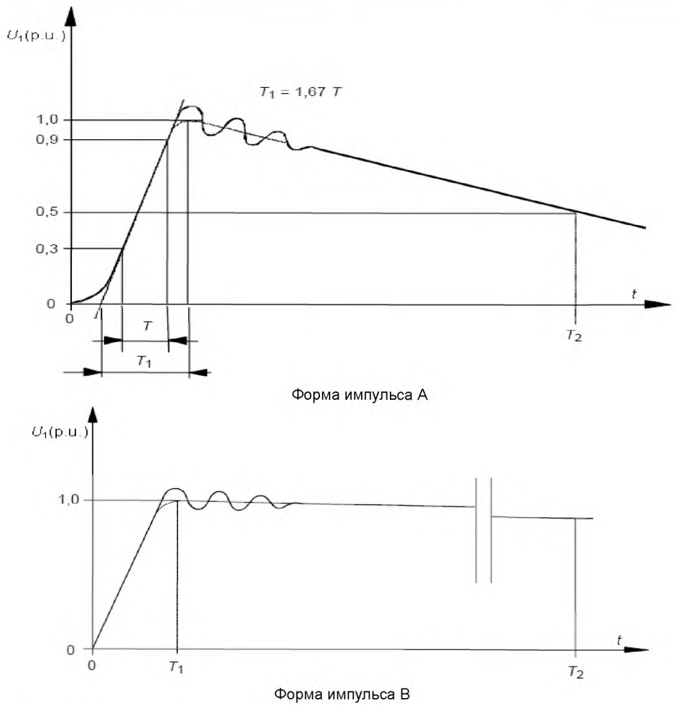
Рисунок 3 — Измерение передаваемых перенапряжений. Форма испытательных импульсов
