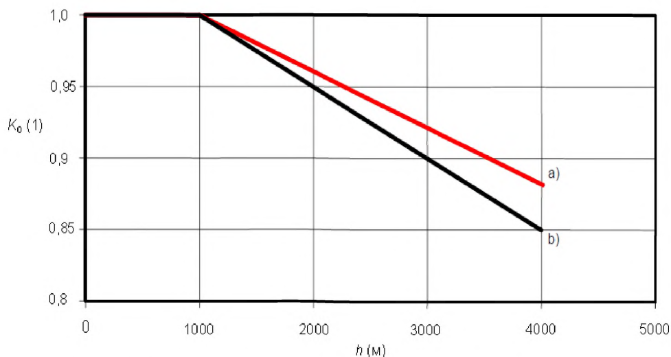
Рисунок 1 — Коэффициент коррекции высоты для превышения температуры
