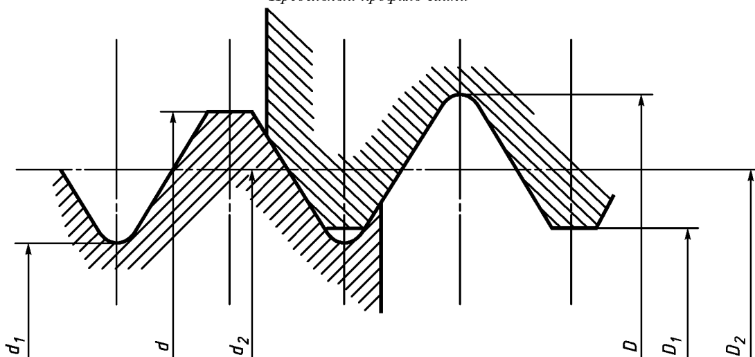
Предельный профиль винта
