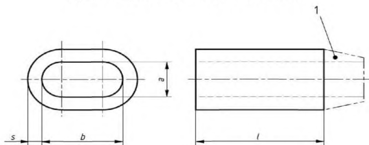
а) Цилиндрическое кольцо типов А и В
