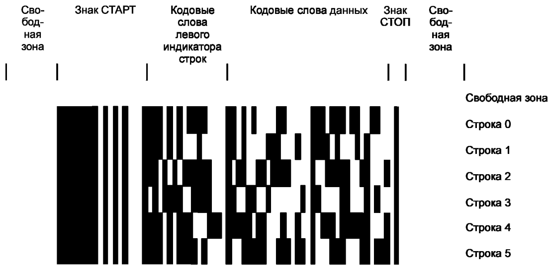
Рисунок G.1 — Компакт PDF417
