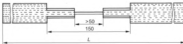
Рисунок 3 — Образец типа В
