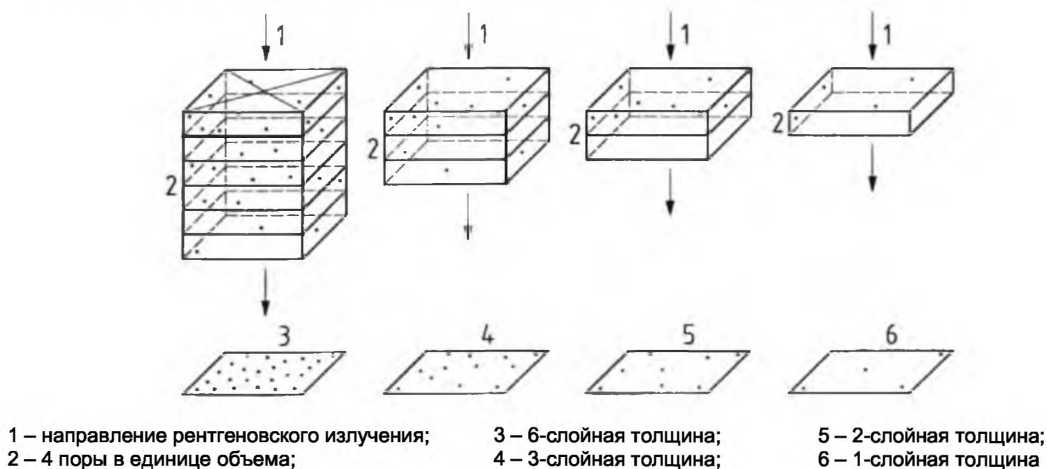
Рисунок 1 – Радиографические снимки образцов с идентичным местоположением пор в единице объема
