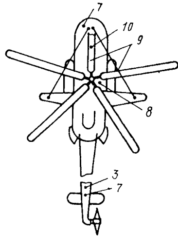
Рис. 18. Размещение излучающих антенн радиотехнических устройств на вертолете Ми-6:
