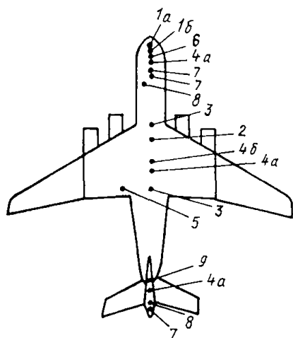
Рис. 2. Размещение излучающих антенн радиотехнических устройств на самолете Ил-76: 1а - КП-2В-5 (РЛС-П); 1б - КП-3А (РЛС-Н); 2 - ДИСС-013-С2 (ДИСС-ЗП); 3 - РВ-5; 4а - СОМ-64; 4б - СО-70; 5 - СДК-67; 6 - РСБН-7С; 7 - И-020; 8 - Баклан-20; 9 - Микрон (ядро)
