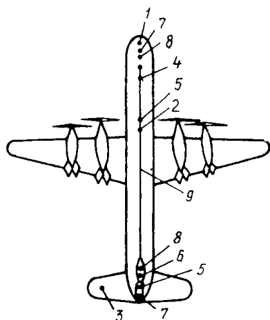
Рис. 4. Размещение излучающих антенн радиотехнических устройств на самолете Ил-18:
