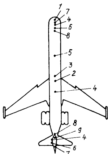
Рис. 3. Размещение излучающих антенн радиотехнических устройств на самолете Ил-62:
