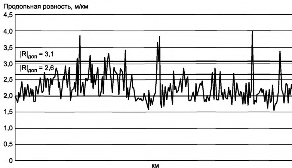
Рисунок А.7 — Продольная ровность покрытия нежесткой дорожной одежды, замеренная на участке по внутренней полосе движения в обратном направлении (полоса б)
