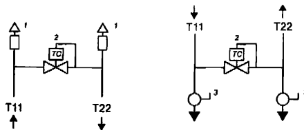
Рисунок 7.3 – Схема КТП, укомплектованного термическим мостом циркуляции
