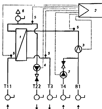
Рисунок 7.13 – Гидравлическая схема КТП для обеспечения локального ГВС
