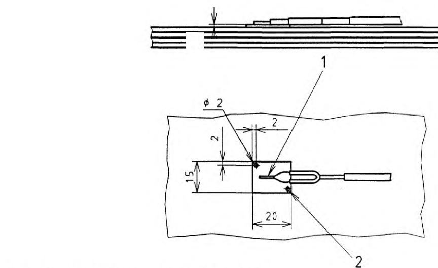
Рисунок 1d – Размещение термопар для измерения температуры испытательных панелей и пола под котлом (см. 6.3.3)
