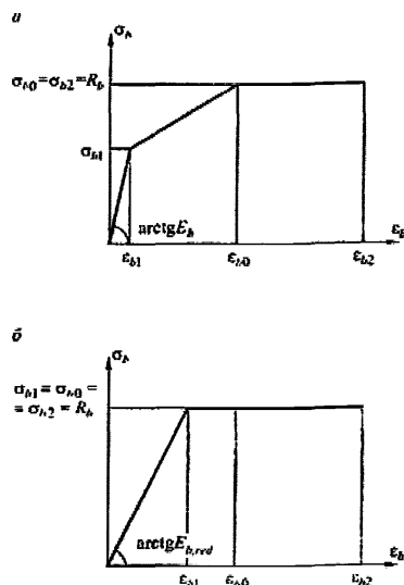
Рисунок 5.1 – Диаграммы состояния сжатого бетона
