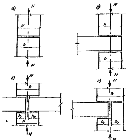
Рисунок В.1 – Опорные сечения стен из панелей (блоков)
