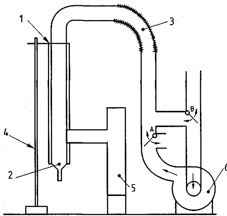
Рисунок 6 – Зонд для отбора проб и положения термопары – Для аппаратов типа С 11
