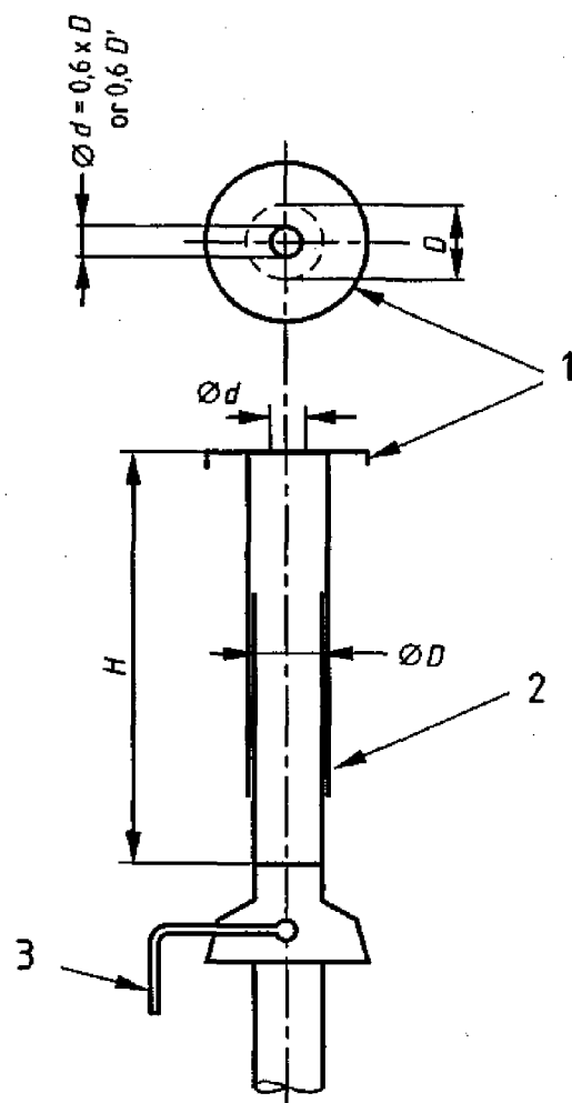
Рисунок 9 – Устройство контроля продуктов сгорания – Испытательная аппаратура (см. 7.9.2.3.2)
