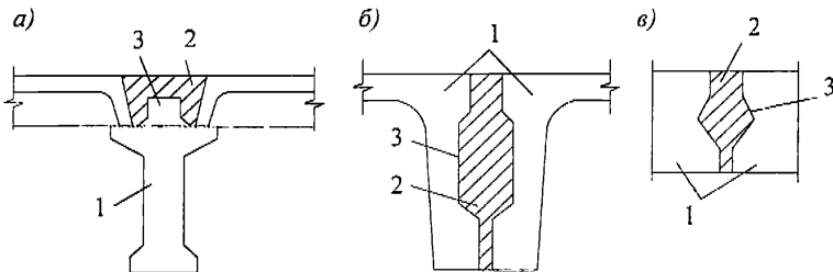
а – ригеля с плитами; б, в – плит между собой; 1 – сборный элемент;
