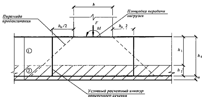
Рисунок 5.15 – Схема для расчета на продавливание при расположении сборного элемента непосредственно под площадкой передачи нагрузки
