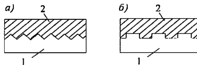
а – треугольные; б – прямоугольные; 1 – сборный элемент; 2 – монолитный бетон
