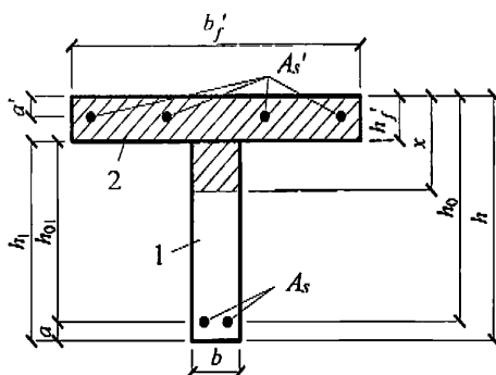
1 – сборный элемент; 2 – монолитный бетон
