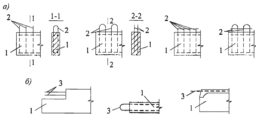
а – поперечная арматура; б – продольная арматура; 1 – сборный элемент; 2 – выпуски поперечной арматуры; 3 – выпуски продольной арматуры
