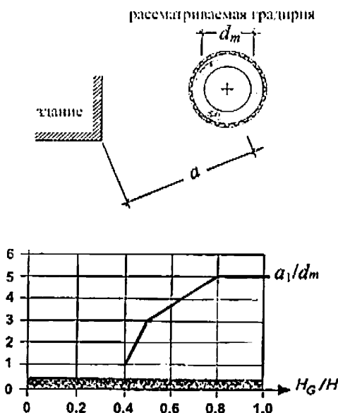
Рисунок Д.4 – Помехи «градирия – здание» в зависимости от отношения H_G/H и верхнего предела a_1/d_m
