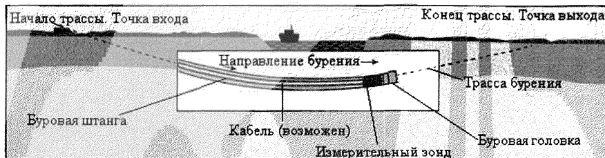
Рисунок 8.3 – Направленное бурение пилотной скважины
