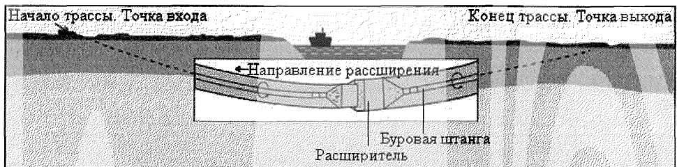
Рисунок 8.4 – Расширение скважины
