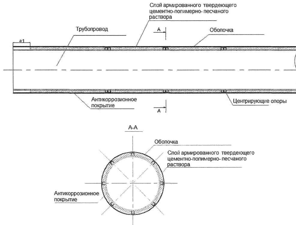
Рисунок Е.1 – Конструкция трубы с ЗКП
