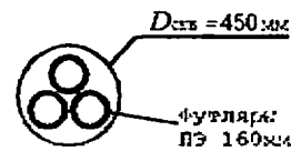
Сечение перехода II-II
