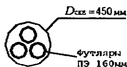
Сечение перехода I-I
