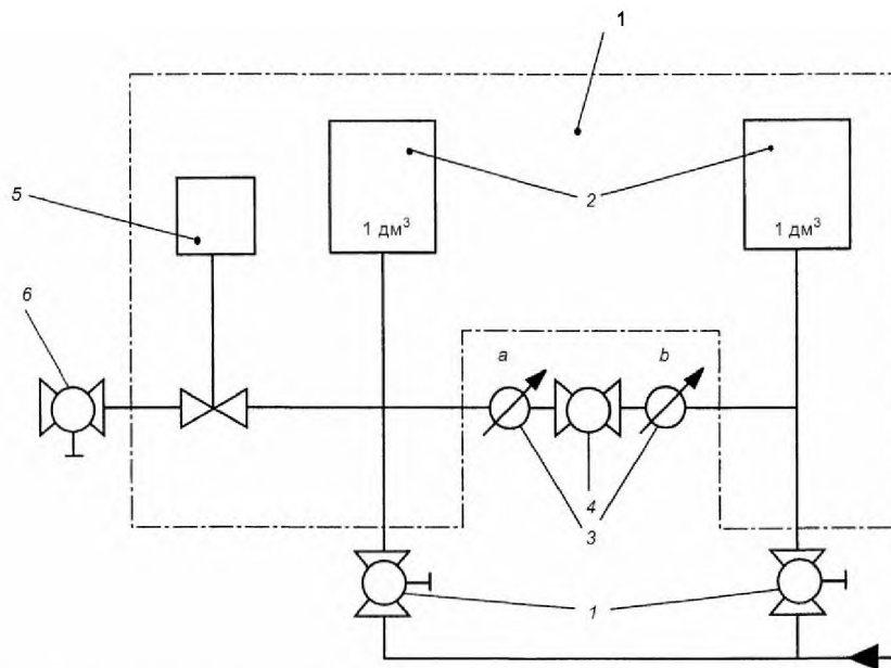
Рисунок 7 – Испытание частей на герметичность (метод потери давления)
