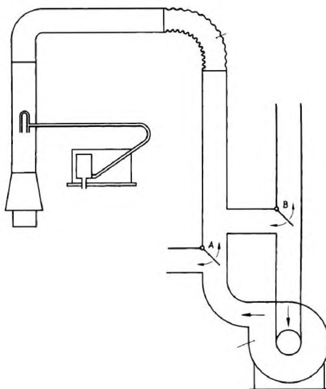
А и В – заслонки для получения восходящей или обратной тяги
