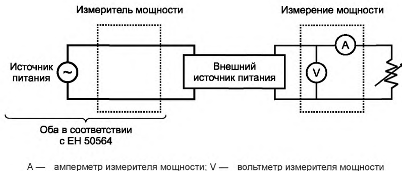
Рисунок 1 — Схема испытания
