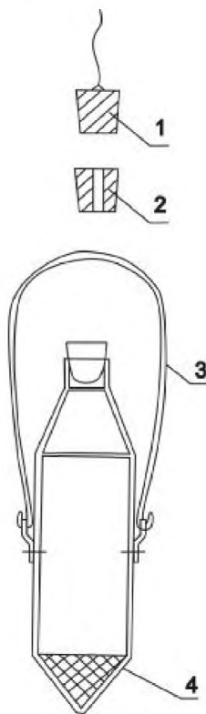
1 – пробка, применяемая при локализованном отборе проб; 2 – пробка, применяемая при непрерывном отборе проб; 3 – металлическая ручка; 4 – свинцовый или бронзовый груз.
