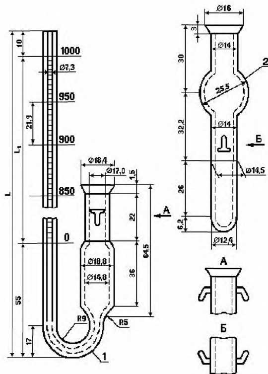
1 – корпус с градуированной трубкой; 2 – пробка
