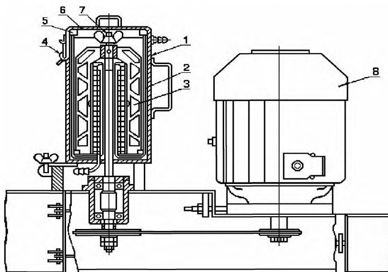
1 – металлический стакан; 2 – рубашка; 3 – мешалка; 4 – зажим; 5 – резиновая прокладка; 6 – крышка; 7 – обогреваемый вал; 8 – электродвигатель
