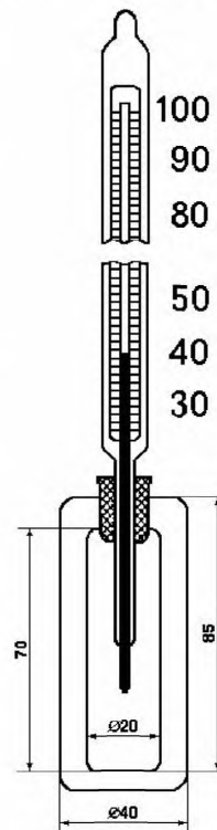
Рисунок 1 – Прибор Жукова
