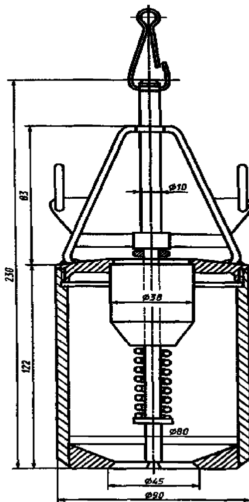
Рисунок А.2 – Зональный пробоотборник
