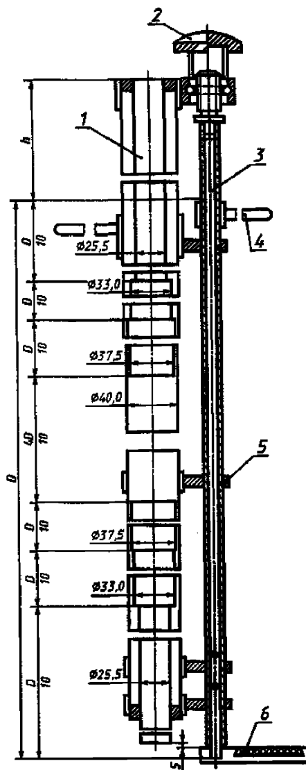
1 – труба; 2 – маховичок; 3 – шток; 4 – рукоятка; 5 – направляющая; 6 – клапан с уплотняющей прокладкой
