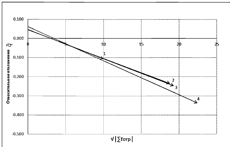
Рисунок И.2 – Зависимость относительных отклонений \tilde{q}_i от корня квадратного из модуля нарастающей суммы отрицательной температуры воздуха для ГП р. Алей – с. Локоть за осенне-зимний период 2005 года
