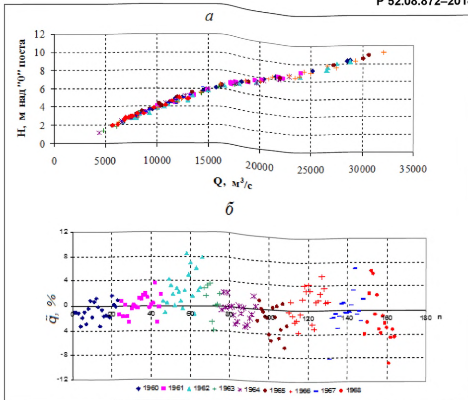
а – МКР Q(H) , б – график относительных остатков регрессии \tilde{q}(n)
