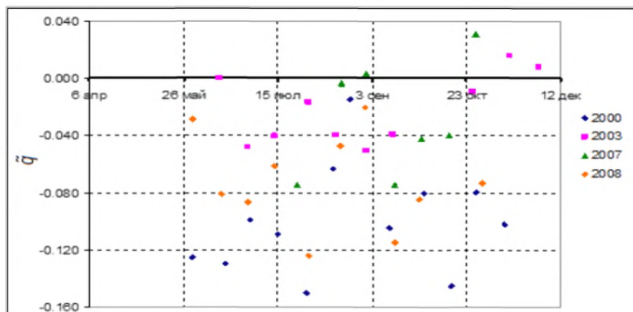
Рисунок 5 – Хронологический график \tilde{q}(t) в период застоя русла, р. Сосна – г. Елец
