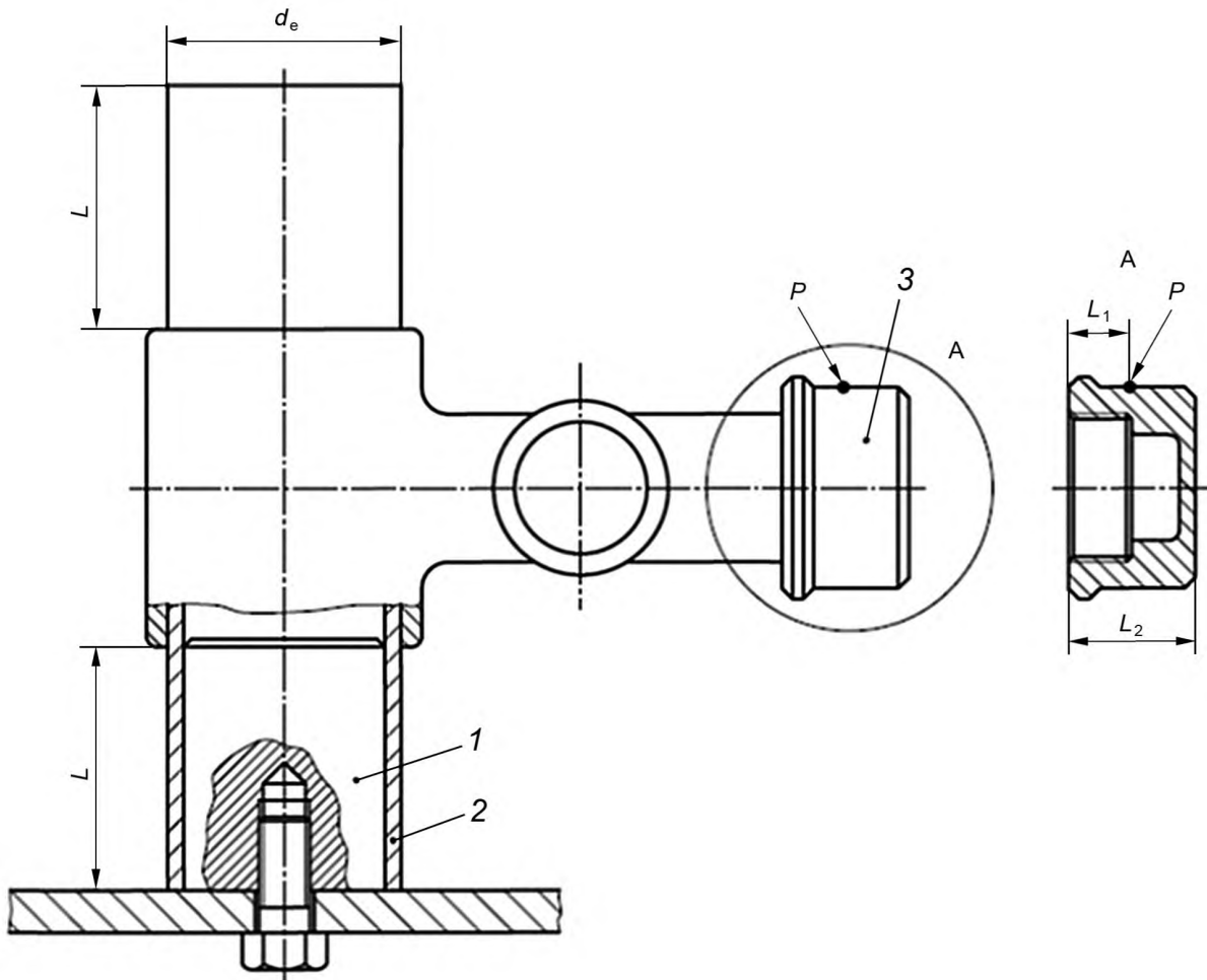
Рисунок ДВ.1 — Образец для испытания
