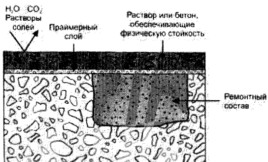
Рисунок Д.3 – Схематичное изображение метода 5.3 до и после применения
