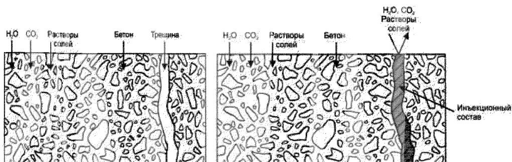
Рисунок А.5 – Схематичное изображение метода 1.5 до и после заполнения трещины
