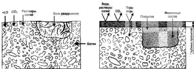
Рисунок Б.3 – Схематическое изображение метода 2.3 до и после устройства покрытия
