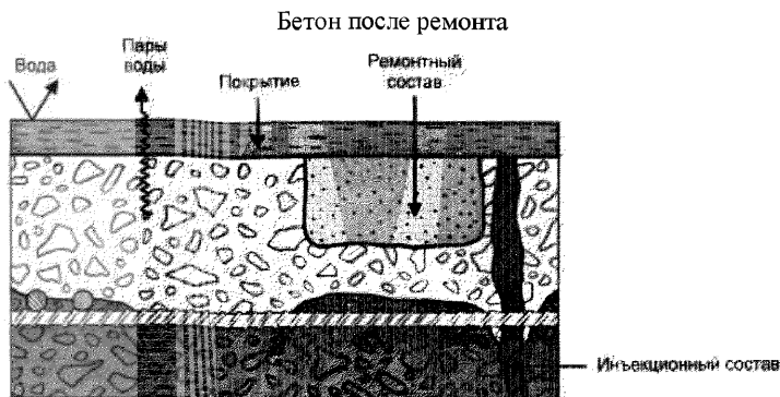
Рисунок И.3 – Схематичное изображение метода 8.3 до и после применения
