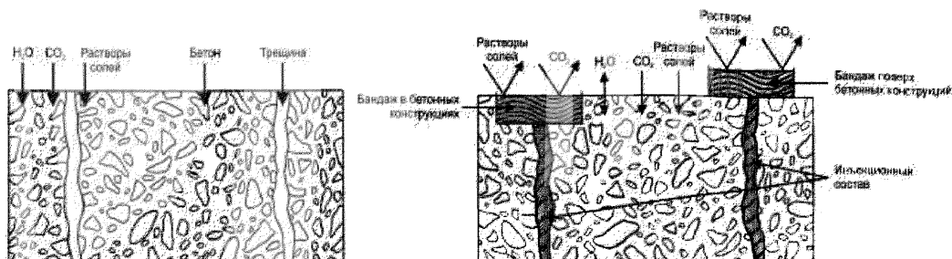
Рисунок А.4 – Схематичное изображение метода 1.4 до и после устройства бандажа
