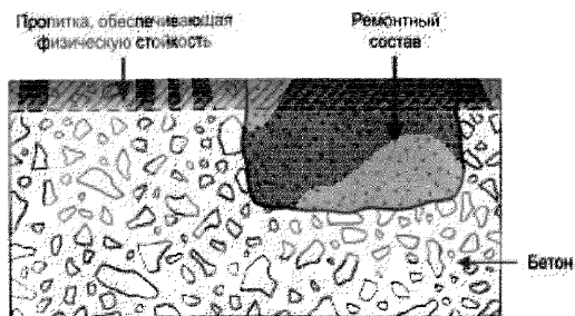
Рисунок Д.2 – Схематичное изображение метода 5.2 до и после применения
