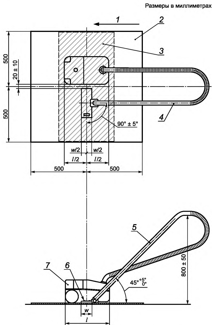
1 — направление ворса; 2 — ковер; 3 — мраморные плиты (при необходимости); 4 — шланг; 5 — трубка; 6 — чистящая головка; 7 — испытуемое изделие; l — длина изделия; w — глубина чистящей головки
