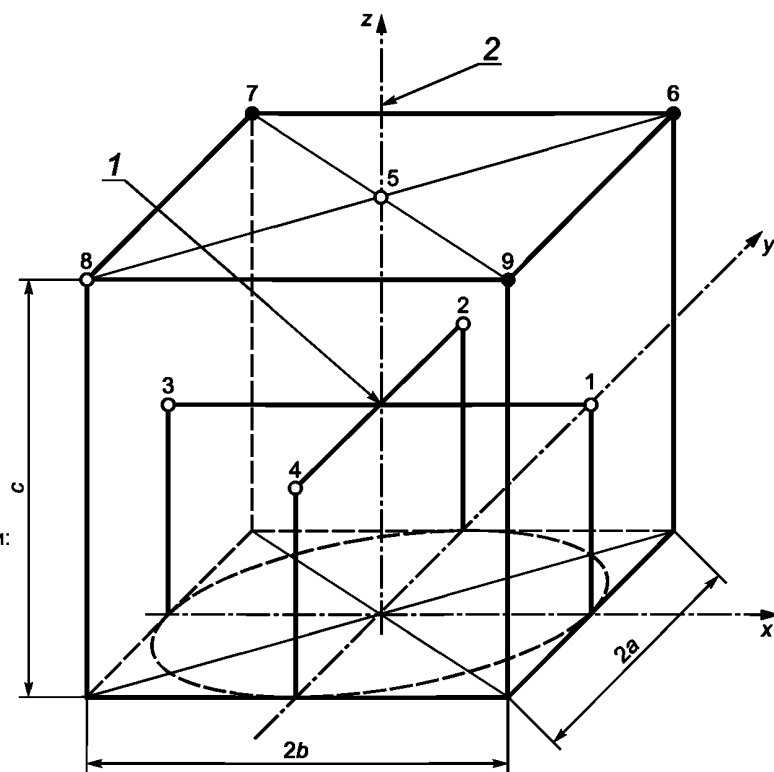
Рисунок 6 — Измерительная поверхность и точки измерений для изделий на стойке (подставке)
