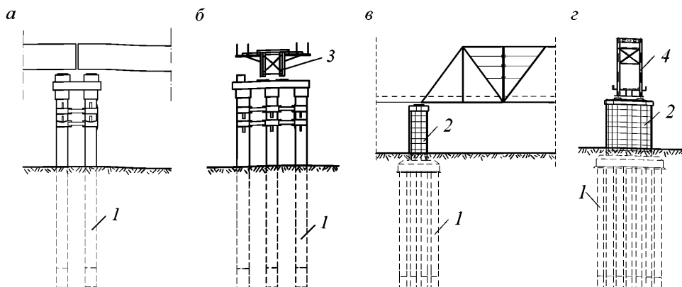
а – столбчатая безростверковая опора, фасад; б – то же, вид вдоль оси моста; в – массивная с высоким ростверком опора, фасад; г – то же, вид вдоль оси моста 1 – столбы; 2 – массивная надфундаментная часть опоры; 3, 4 – пролетные строения соответственно с ездой поверху и понизу
