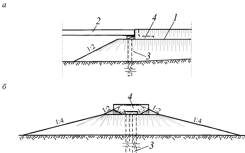
а – фасад оси моста со стороны пролета; б – вид вдоль оси моста со стороны пролета
