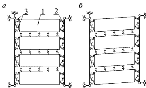
а – расчетная модель ячейки перекрытия; б – схемы деформирования при наличии связей
