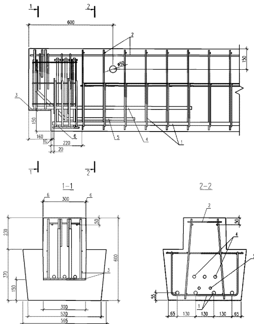
1 – сетка с рабочей арматурой; 2 – пространственный арматурный каркас; 3, 4, 6 – закладное изделие; 5 – отгиб
