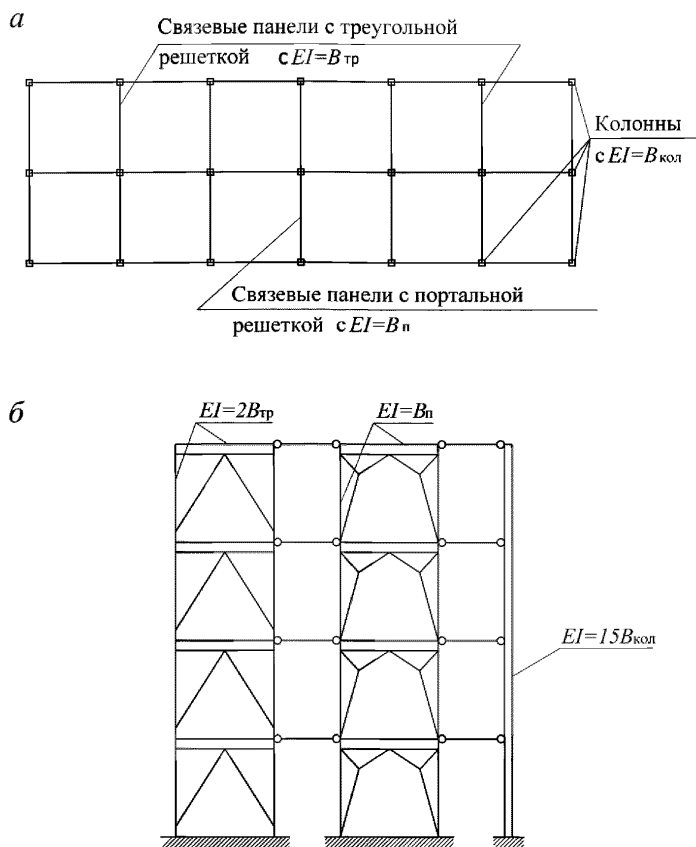
а – конструктивная схема; б – расчетная схема
