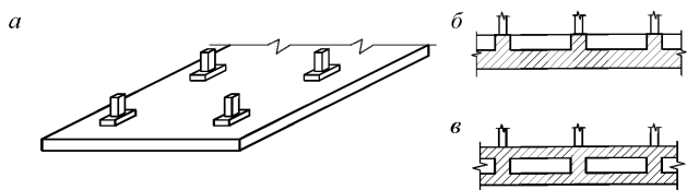
а – плитный безбалочный; б – плитно-балочный; в – коробчатый
