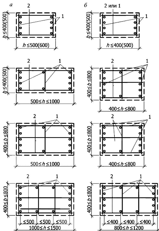
a – колонны, внецентренно сжатых в одной плоскости; б – колонны, внецентренно сжатые в обеих плоскостях; 1 – плоский каркас; 2 – соединительный стержень (поперечный привариваемый стержень или шпилька)
