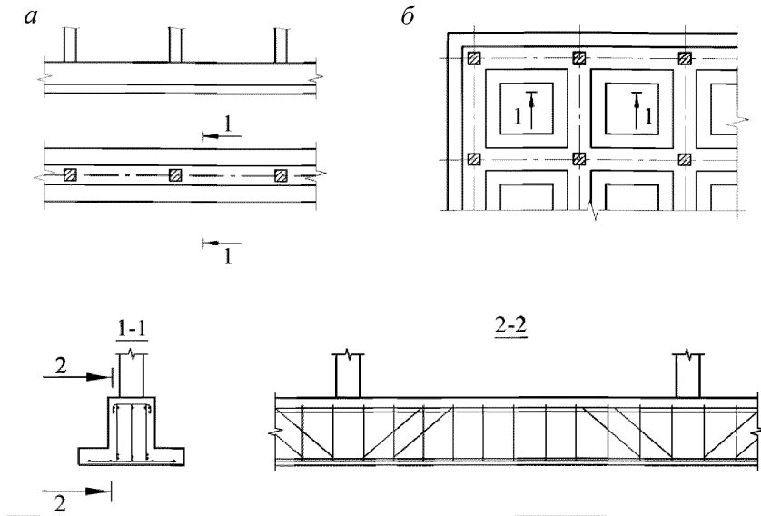
а – отдельные ленты; б – перекрестные ленты
