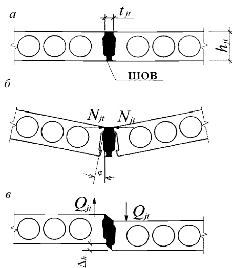
а – схема межплитного шва; б – поворот вдоль продольной оси; в – сдвиг плит
