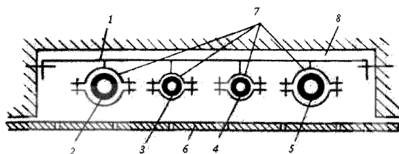
Рисунок 14.4 – Крепление труб из ПЭ-С в штробе
