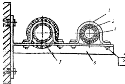
в) Горизонтальные (парные)
