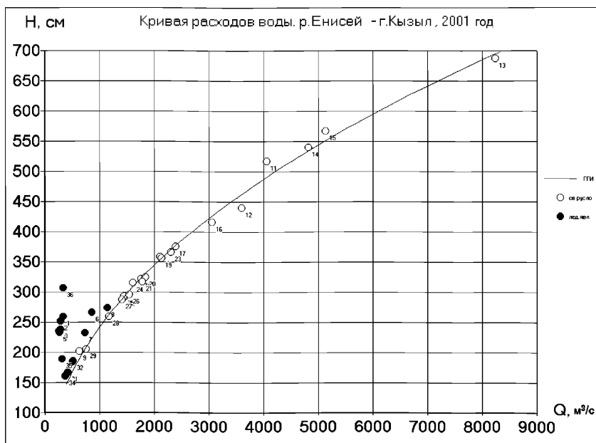
Рисунок А.1 – Зависимость расходов воды от уровней
