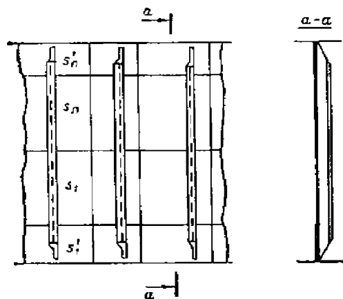
Рис. 2.5.2.3 Конструкция подкрепления обшивки переборок цистерн при обрезке концов балок «на ус»: s'_i = s_i + \Delta_1 ; s'_n = s_n + \Delta_2 ; \Delta_1, \Delta_2 — утолщение поясьев обшивки переборки на концевых участках стоек, срезанных «на ус»
