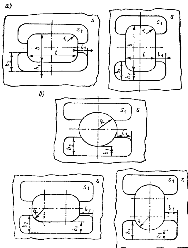
Рис. 1.4.3.3 Подкрепление прямоугольных (а), круглых и овальных (б) вырезв в бортах утолщенными сварными листами
