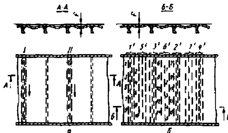
Рис. 6.5.1.1-1 Схема правки конструкций с ребристостью:
