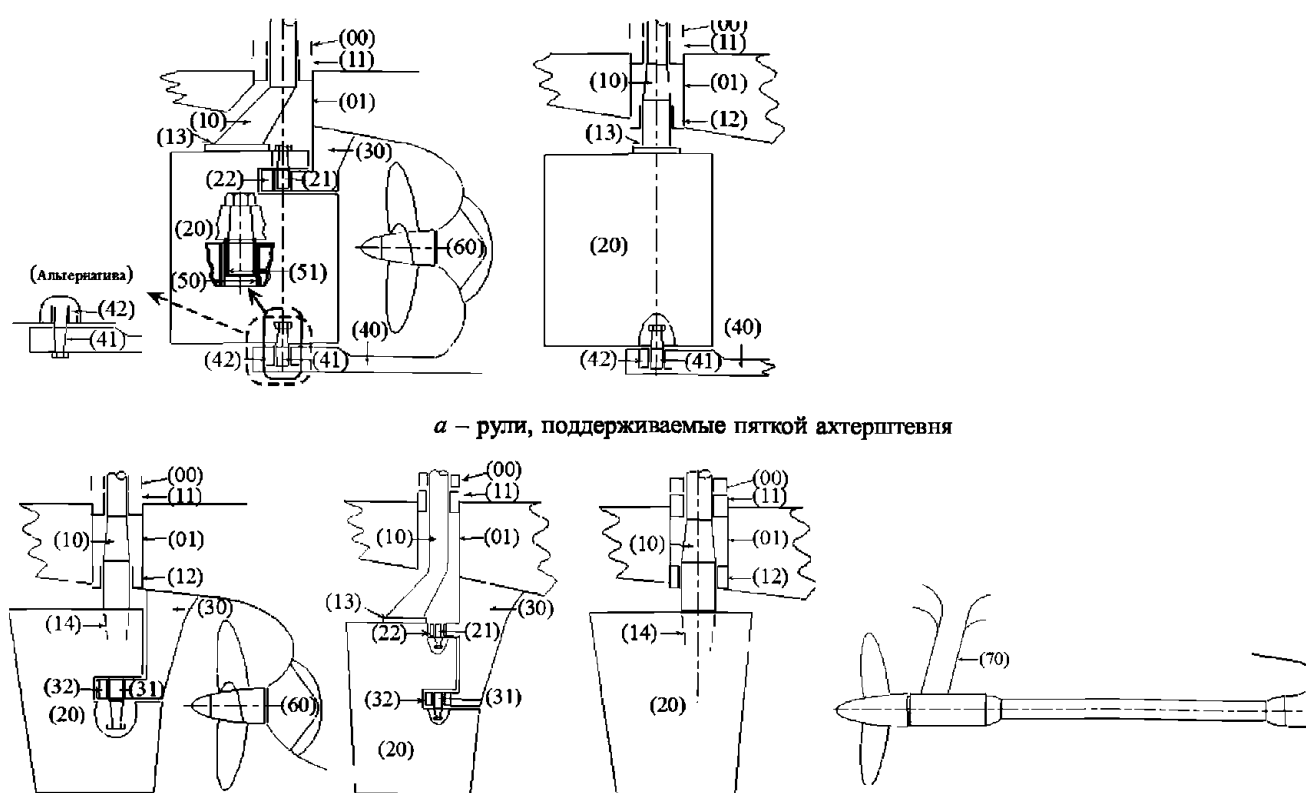
а – рули, поддерживаемые пяткой ахтерштевня; б – рули полулопатообразной формы; в – руль лопатообразной формы; г – устройство опоры для двух винтов
