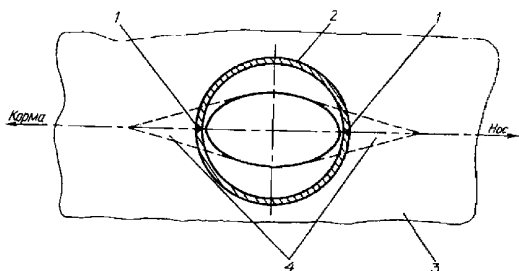
Рис. 1.4.2.6.3 Расположение стыковых швов в районах круглых (эллиптических) вырезом: 1 — стык; 2 — комингс шахты; 3 — палуба; 4 — неэффективный участок
