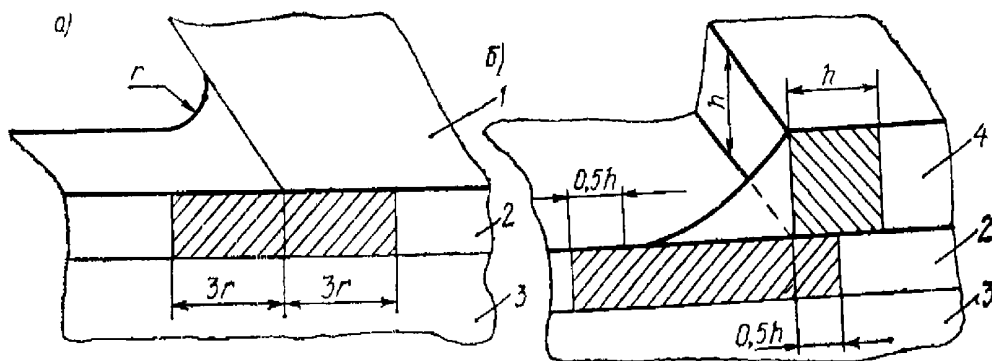
Рис. 1.4.3.7 Особые участки подкреплений вырезов в ширстрек:
