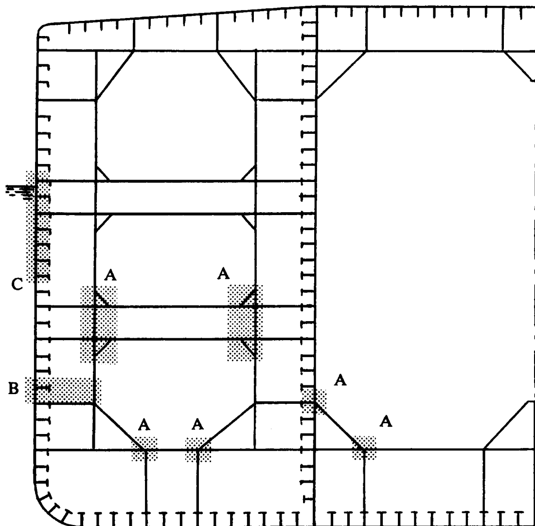
Рис. 2.1-7 Районы концентрации напряжений в элементах корпуса нефтеналивного судна:
