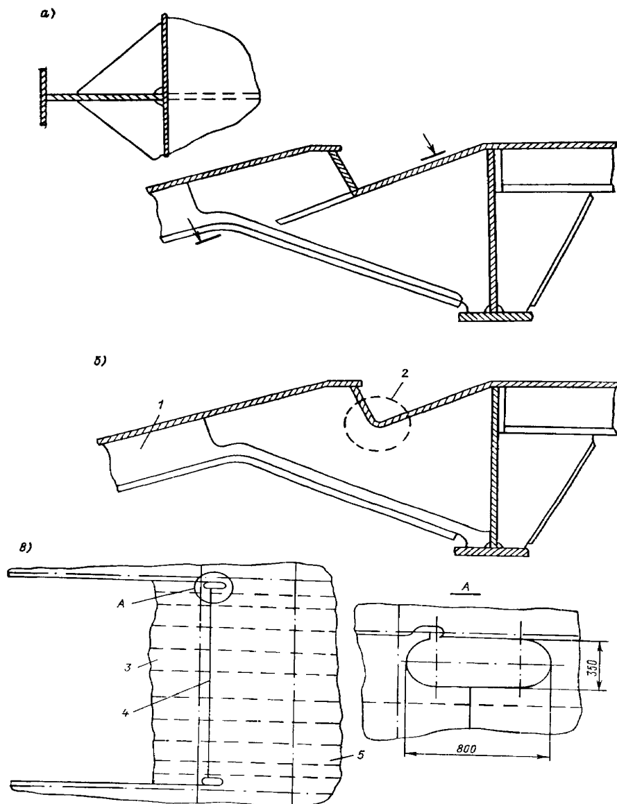
Рис. 2.4.18.3 Узел соединения съездной рампы с палубой (а), скругление настила палубы по дуге малого радиуса (б) и переход настила верхней палубы (второго дна) в настил наклонного съезда (в):
