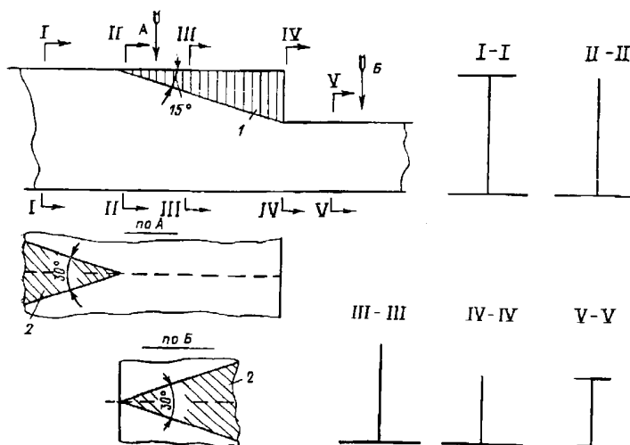
Рис. 2.2.3.8.1 Неэффективные участки флора в районе уступа двойного дна: 1 — неэффективный участок стенки флора (см. рис. 1.1.2, б); 2 — присоединенный пояс; I — I ... V — V — расчетные сечения с учетом изменения присоединенного пояска
