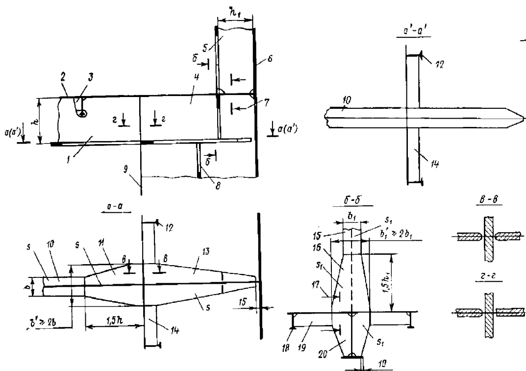
Рис. 2.3.10.2 Соединения рамных шпангоутов в твиндеке с палубой над двойным бортом на накатных судах (судах ро-ро):
