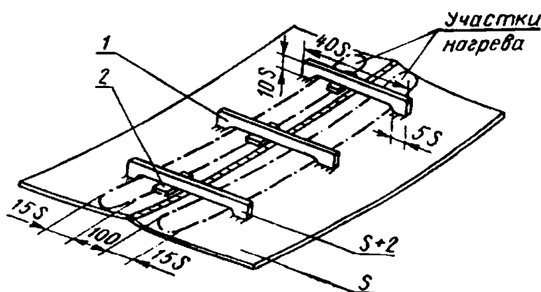
Рис. 6.4.1 Схема нагрева обшивки при правке методом низкотемпературного нагрева:
