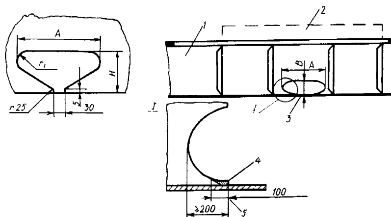
Рис. 2.4.10.6 Отверстия для пропуска воды в стенках непрерывных комингсов (в районе между смежными поперечными комингсами):
