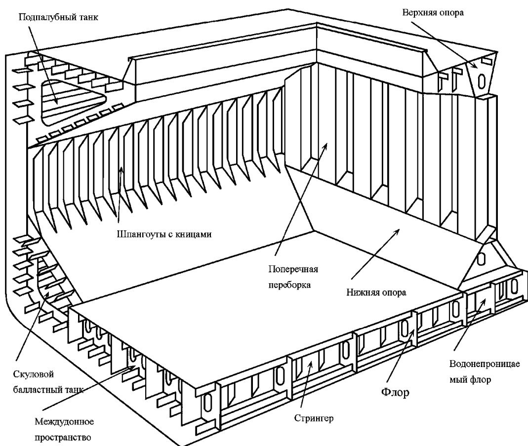
Рис. 1-3 Типовая схема грузового трюма навалочного судна с одинарной обшивкой
