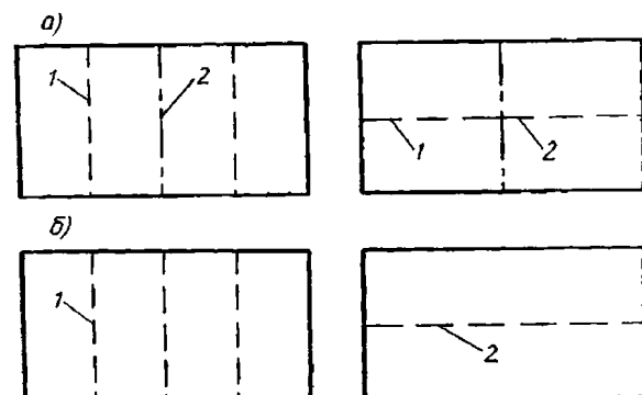
Рис. 2.2.3.5.3 Подкрепление стенок вертикального киля (а) и днищевого стрингера (б):
