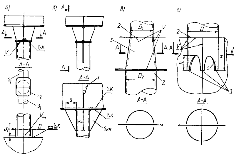
Рис. 2.4.8.1 Конструкции закрепления верхних и нижних концов пиллерсов:
