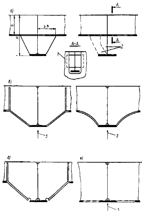
Рис. 2.4.7 Соединения рамных бимсов с карлингсами:
