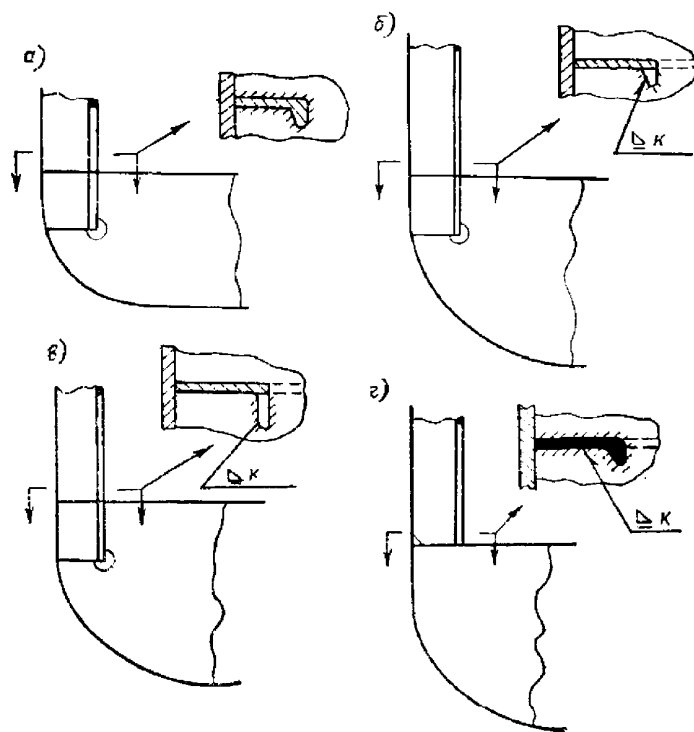
Рис. 2.3.1.4 Бескнижное соединение шпангоута с двойным дном:
