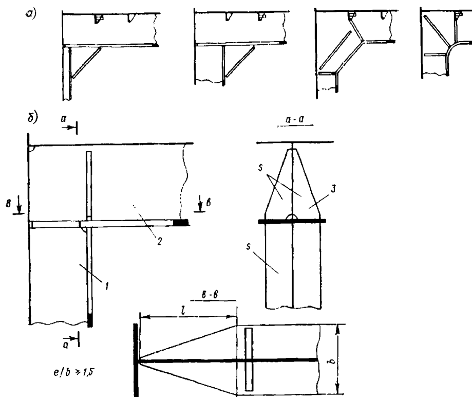
Рис. 2.4.6.1 Соединения рамных бимсов с основными и рамными шпангоутами:
