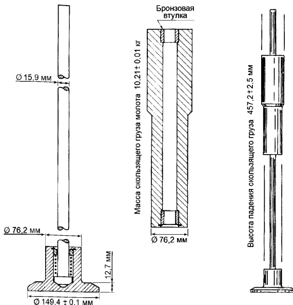
Рисунок 4. Уплотнительный молот
