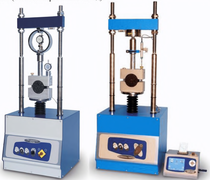
Рисунок 1. Типовое оборудование по методам А и Б
