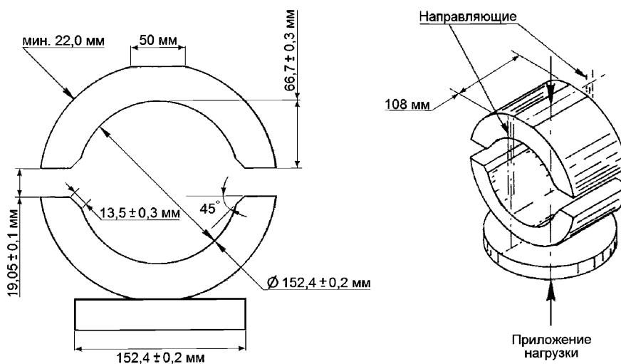
Рисунок 6. Типовая обжимная головка
