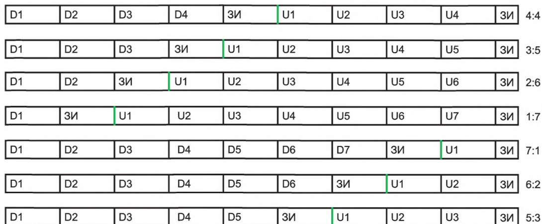
Рисунок 18 — Распределение тайм-слотов в радиополосах DL/UL для кадра длительностью 10 мс
