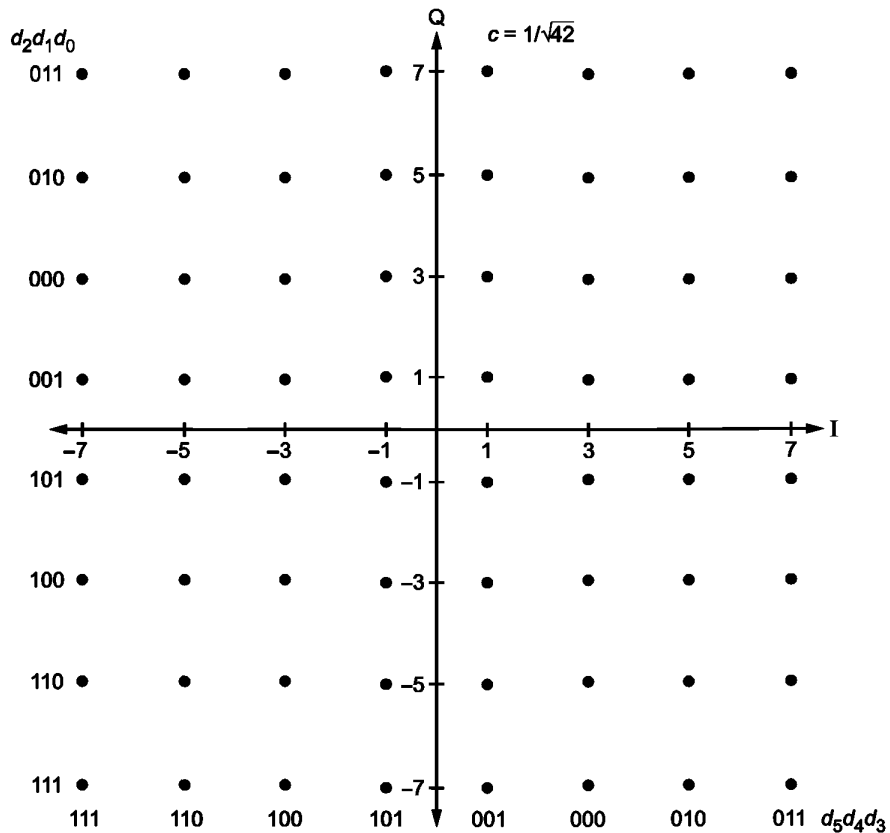
Рисунок 7 — Созвездие 64QAM
