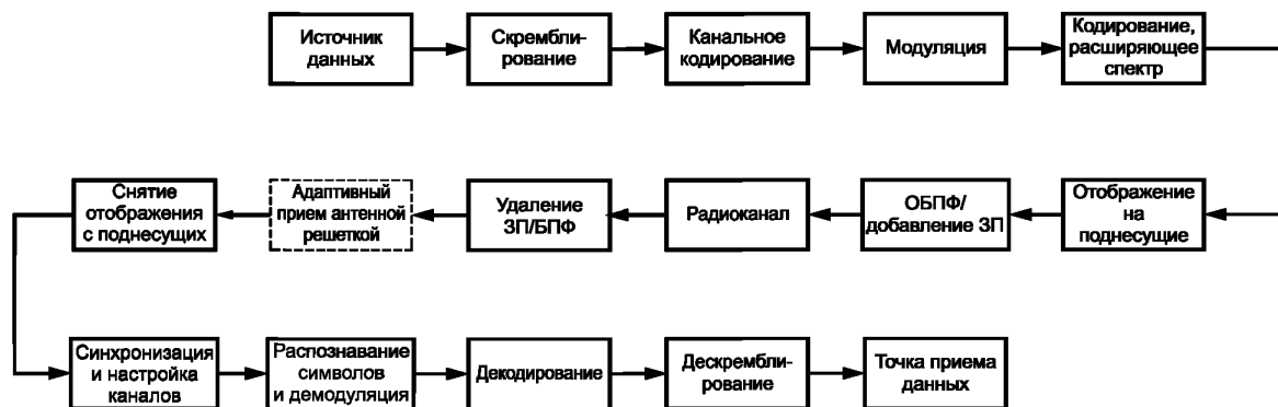
Рисунок 3 — Преобразование потока данных в радиолинии UL
