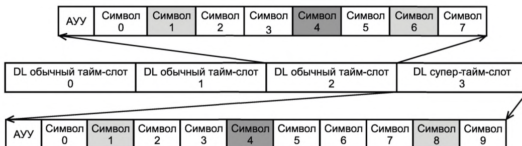
Рисунок 14 — Структура тайм-слотов в кадре трафика в DL длительностью 10 мс
