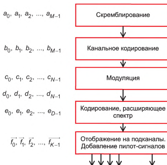
Рисунок 1 — Диаграмма преобразования потока информации на физическом уровне
