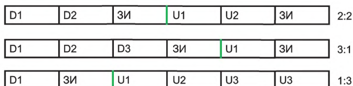
Рисунок 19 — Распределение тайм-слотов в радиополосах DL/UL для кадра длительностью 5 мс
