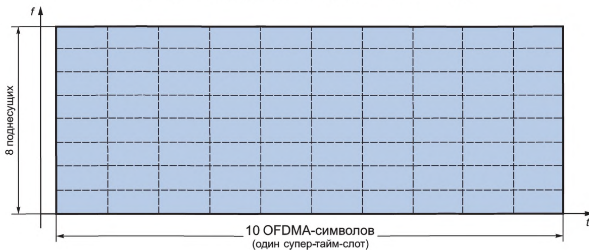
Рисунок 21 — Структура подканала (ПдК) в супер-тайм-слоте
