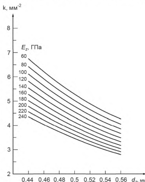
Рисунок 2 — Диаграмма для определения коэффициента k как функции толщины цирконовой подложки d_z и модуля Юнга E_z диоксида циркония
