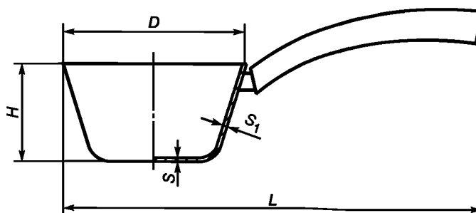
Рисунок 7 — Ковш
