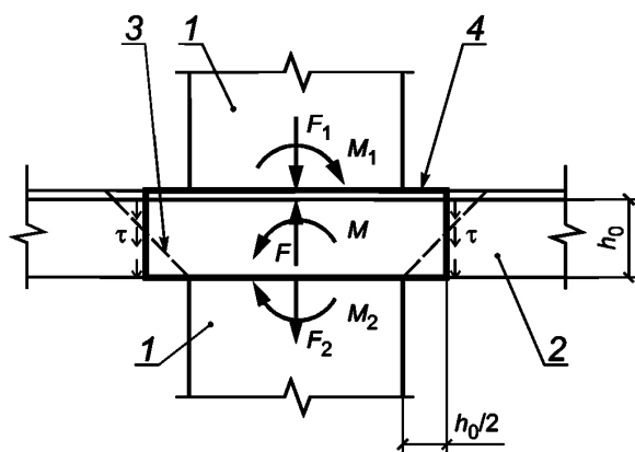
1 — колонна; 2 — плита; 3 — пирамида продавливания; 4 — условный расчетный контур
