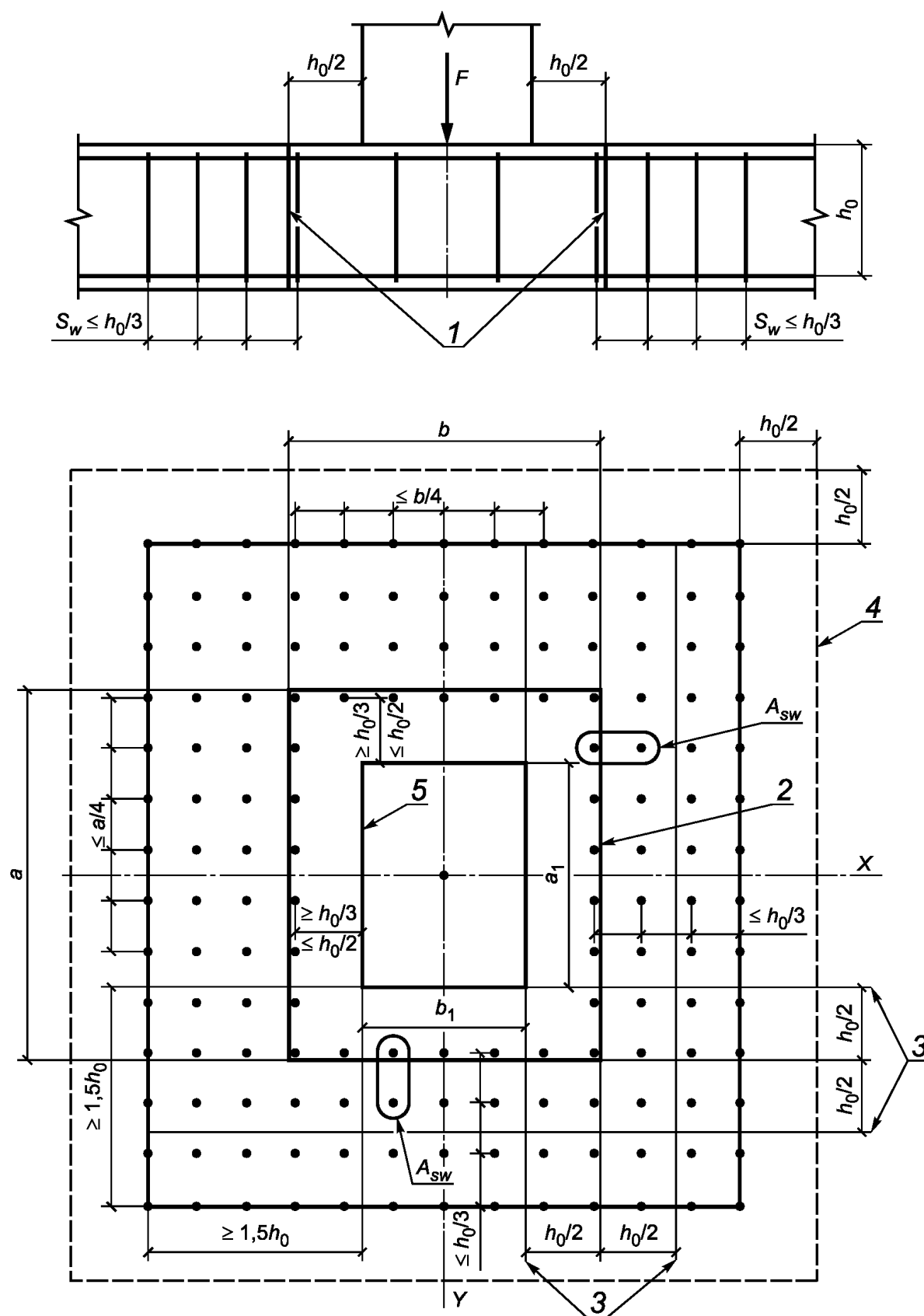
Рисунок 18 — Схема для расчета сталефибробетонных плит с вертикальной равномерно распределенной поперечной арматурой на продавливание
