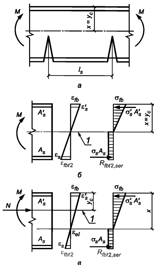
Рисунок 20 — Схема напряженно-деформированного состояния элемента с трещинами при действии изгибающего момента (а, б), изгибающего момента и продольной силы (в)
