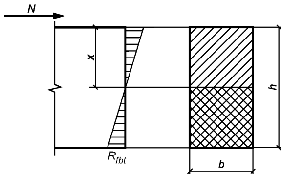
Рисунок 8 — Схема усилий и эпюра напряжений в сечении, нормальном к продольной оси внецентренно сжатого сталефибробетонного элемента, рассчитываемого по прочности с учетом сопротивления сталефибробетона растянутой зоны
