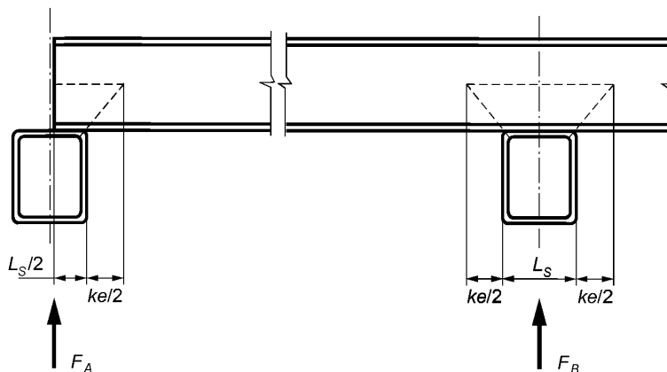
Рисунок 9 — Призма смятия утеплителя сердцевинки над опорой
