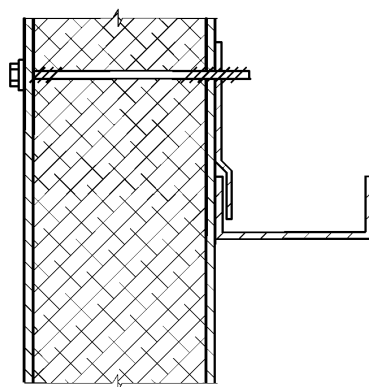
Рисунок 11 — Крепление панели к каркасу в холодильниках
