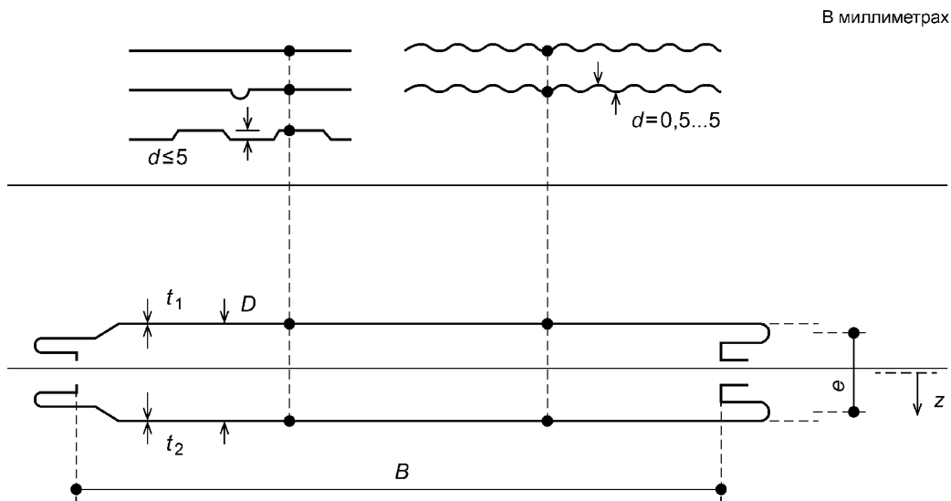
Рисунок 1 — Параметры гладких и слабопрофилированных обшивок
