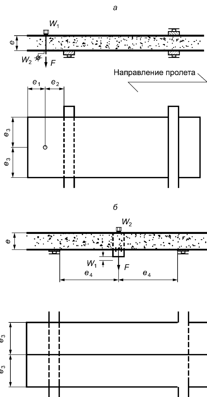
a — крепление на крайней опоре; b — крепление на средней опоре; e_1 — минимальное расстояние от кромки панели; e_2 \geq 100 мм; e_3 \geq B/4 ; B — ширина панели; e_4 \geq 100 мм
