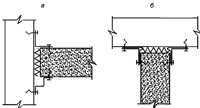
а — потолок — внешняя стена; б — внутренняя стена — потолок (эластичной лентой); в — внутренняя стена — потолок; а — внутренняя стена — внешняя стена (вариант)
