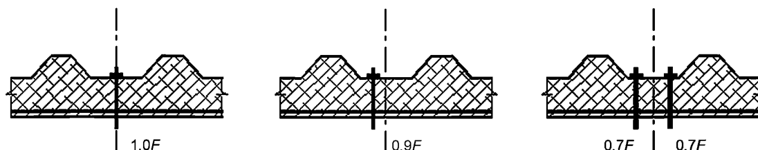
Рисунок 12 — Крепление кровельных панелей самонарезающими винтами
