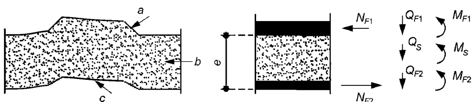
Рисунок 5 — Схема внутренних усилий в сечении панели с профилированными обшивками
