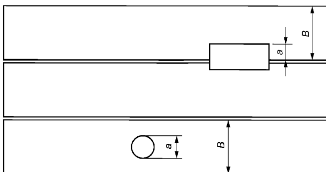
Рисунок 13 — Влияние небольших отверстий на несущую способность панелей
