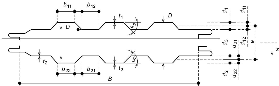
Рисунок 2 — Параметры профилированных обшивок
