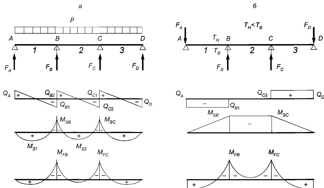
а — усилия в панели от постоянной нагрузки; б — усилия в панели от разности температур на обшивках; 1, 2, 3 — пролеты Рисунок 8 — Эпюры M и Q в трехслойных панелях и их обшивках от поперечной равномерно распределенной нагрузки и разности температур на обшивках панели
