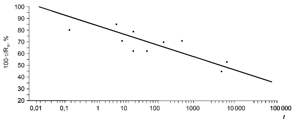
Рисунок 15 — Пример прямолинейной регрессии
