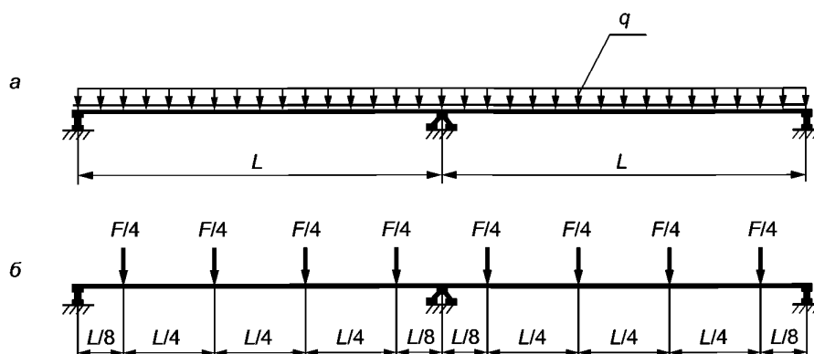
а — при использовании надувного воздушного мешка или вакуумной камеры; б — при использовании сосредоточенных линейных нагрузок, создаваемых гидравлическими домкратами
